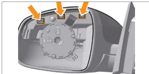
Рис. 8.18. Защелки накладки зеркала
