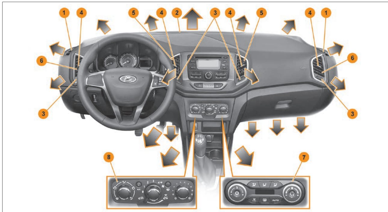
Рис. 6.1. Климатическая система
